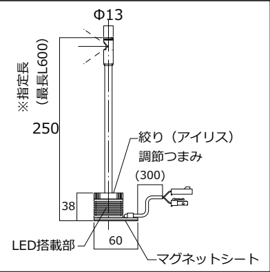
10° 25° 10~45 ※指定長（最長L600） 250 38 60 LED搭載部 絞り（アイリス） 調節つまみ (300) マグネットシート
